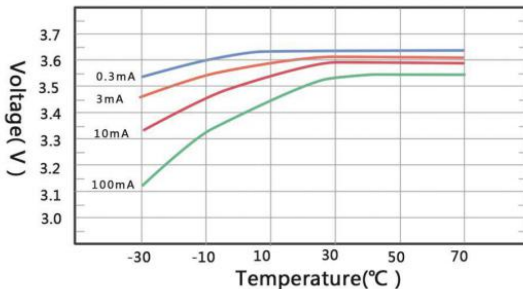
不同温度下电压平台特性图
