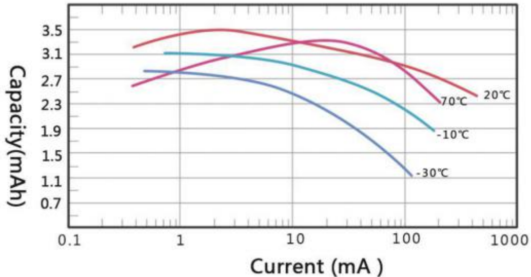
不同放电电流与放电容量特性图
