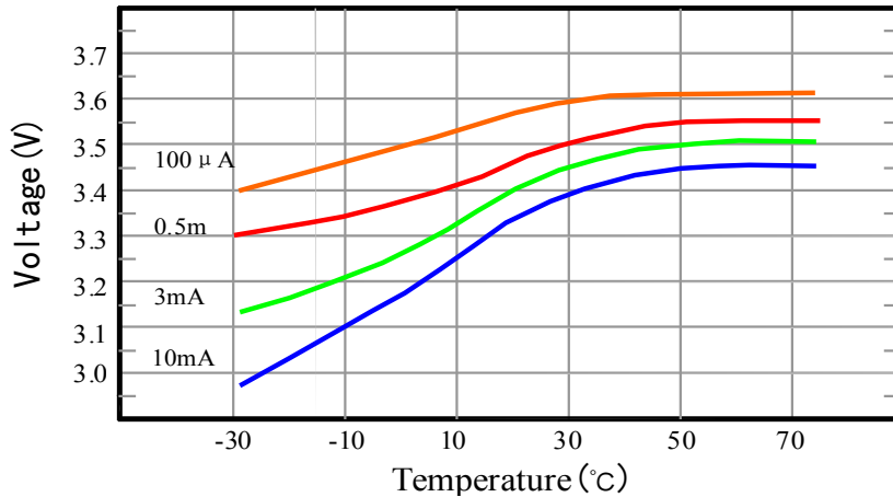
不同温度下电压平台特性图
